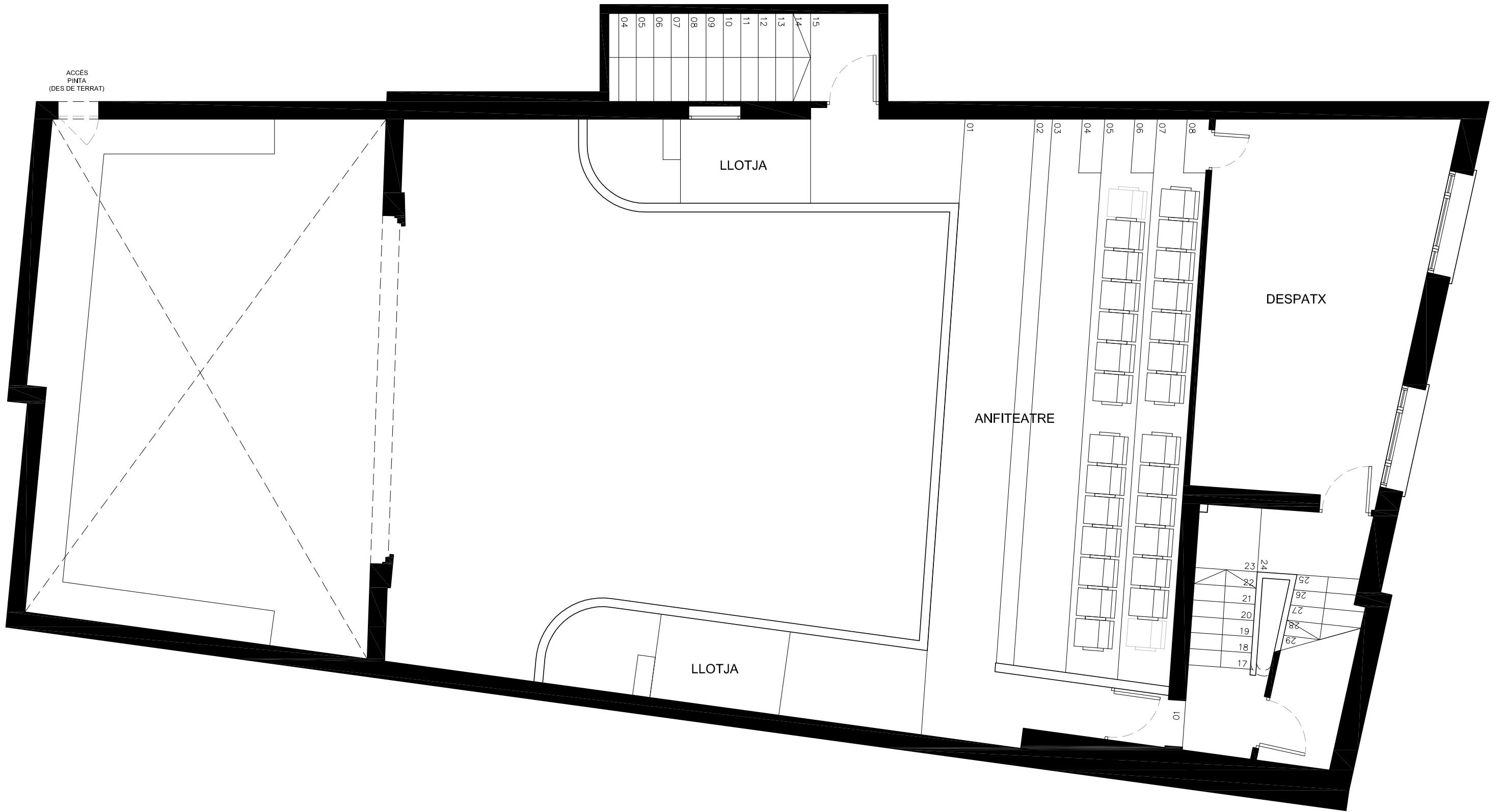
PLANTA ANFITEATRE 26 BUTAQUES
